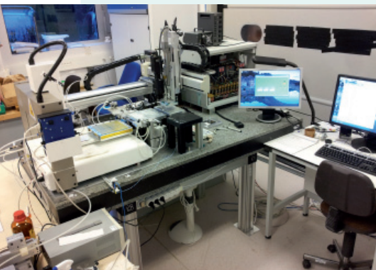
Robot de positionnement et de collage de capteurs silicium sur des cartes électroniques.
