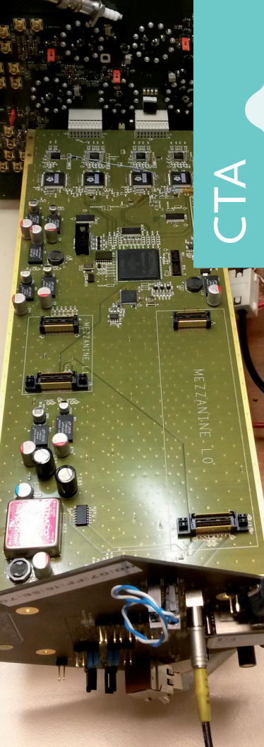
Carte de lecture d'un module de détection NECTAR.
