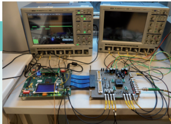
Banc de test modulaire (ici, pour le circuit CABAC1).
